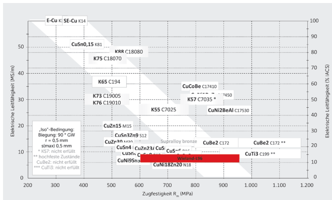
Position des L96 im Leitfähigkeits-Festigkeits-Diagramm
