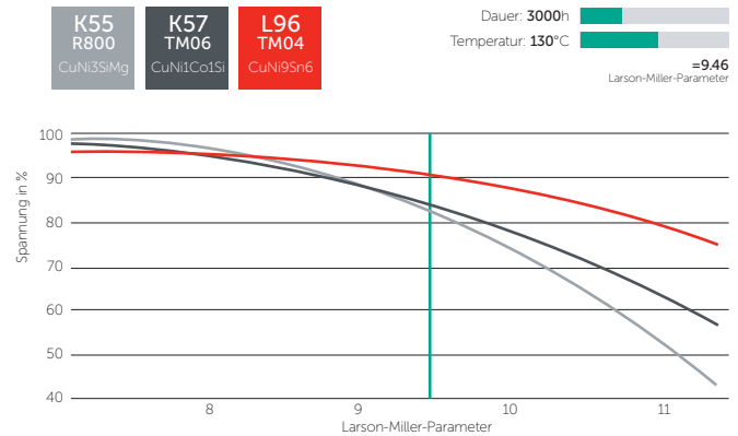
Thermische Spannungsrelaxation von L96 TM04 im Vergleich zu K55 R800 und K57 TM06
